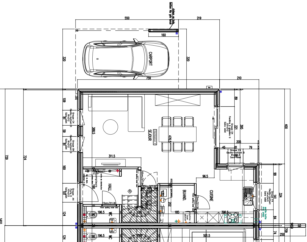
-REZ-de-CHAUSSEÉ- 62,28m 2 + carport 17,62m 2 PAS 0 LOT 4
