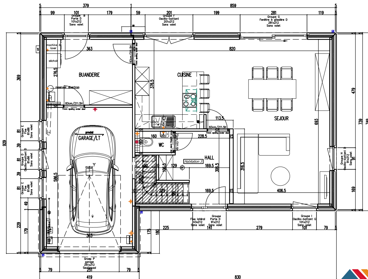
-REZ-de-CHAUSSEE- 101,08m 2 PAS 0 LOT 3
