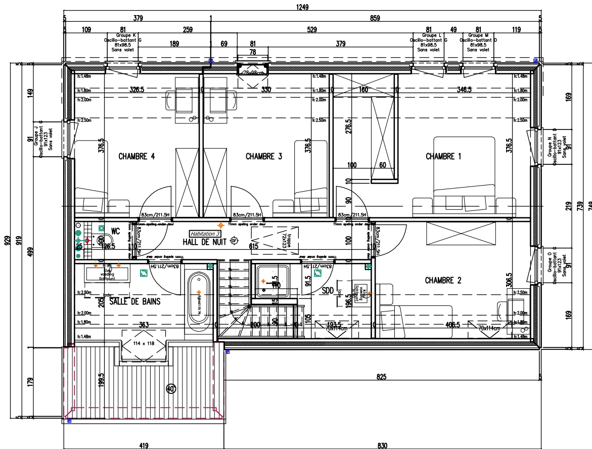
-ETAGE- 92,82m 2 PAS 287 LOT 3
